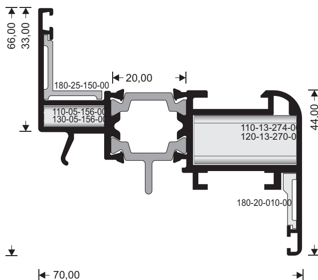
KRILO MALO-RAVNO SASH SMALL FLAT
