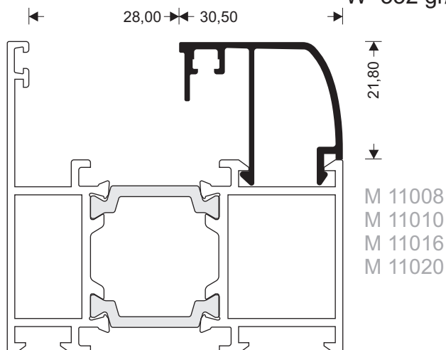
LAJSNA ZA STAKLO GLAZING BEAD
